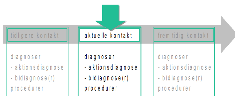
Figur 2 Kontaktmodellen
